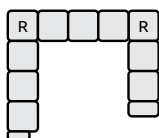
Helix B-3Rm-ROH-3Sp-ROH-2Su-PT 340 × 99 × 266/254 cm včetně R + ÚP
